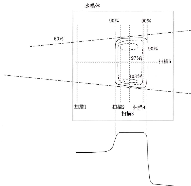
图 4 测量横向剖面曲线的深度
