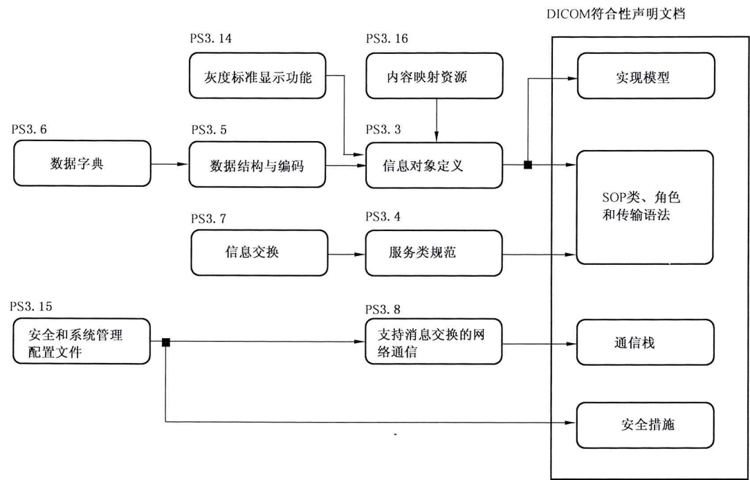
图 A.1 网络符合性声明的构建过程
