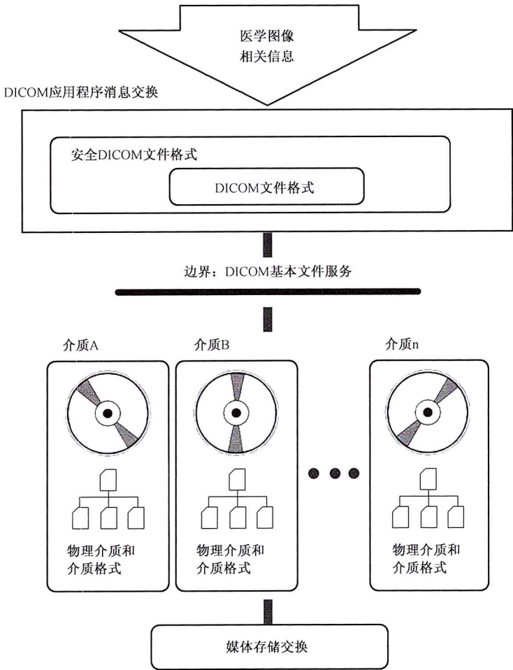
图 A.3 DICOM 媒介通信模式
