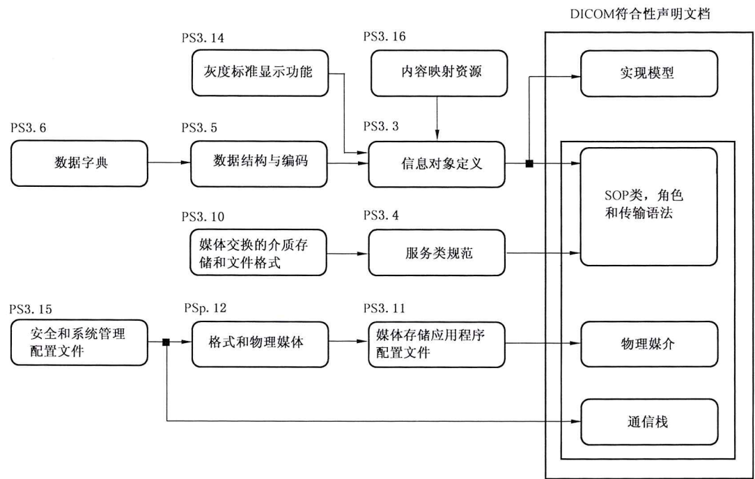
图 A.2 媒介符合性声明的构建过程
