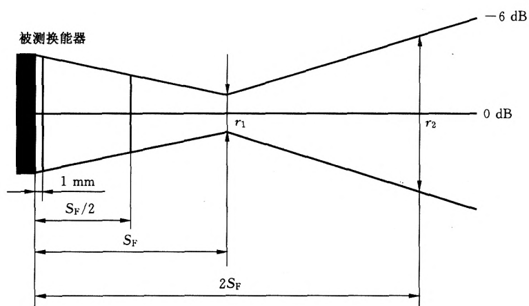
图 12 聚焦换能器声场中四个位置的波束宽度几何图
