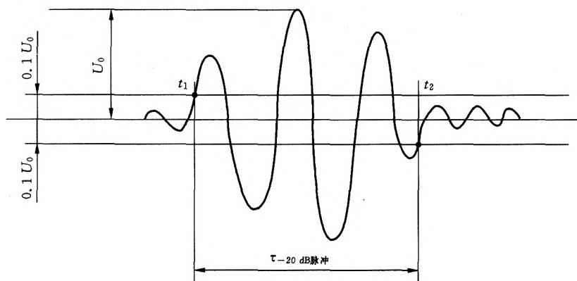
图8 -20 dB 脉冲宽度波形图
