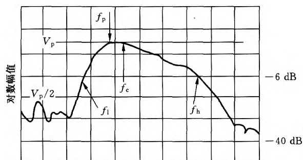
图 4 频率-振幅谱的标绘图
