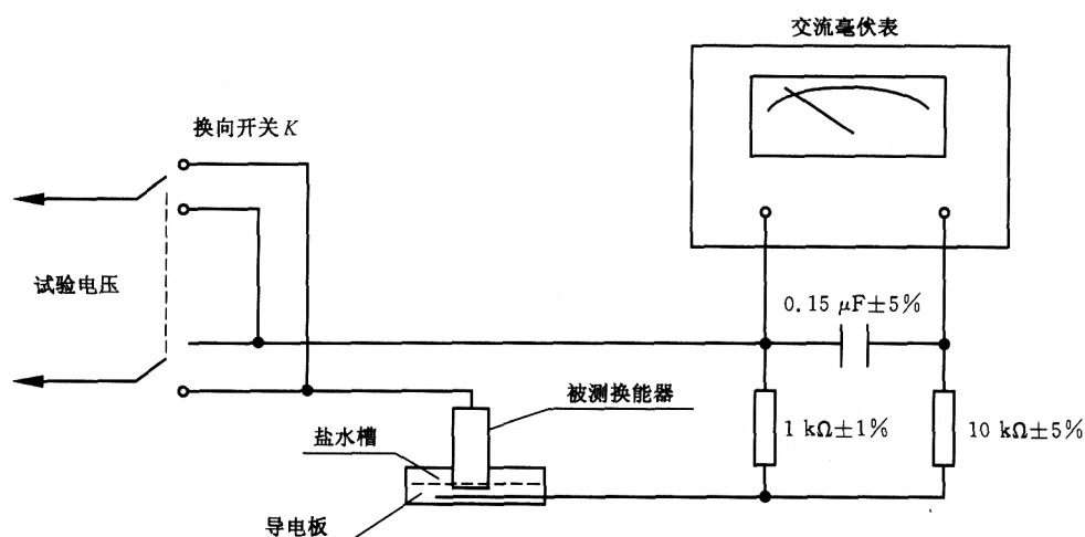
图 15 测量换能器介电绝缘性的原理图
