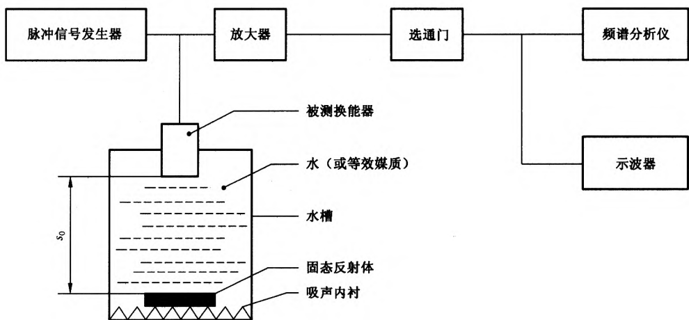
图 6 频谱法工作原理图
