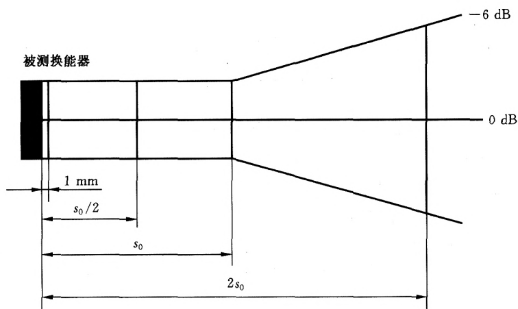
图 11 被测换能器声场中四个位置的波束宽度几何图
