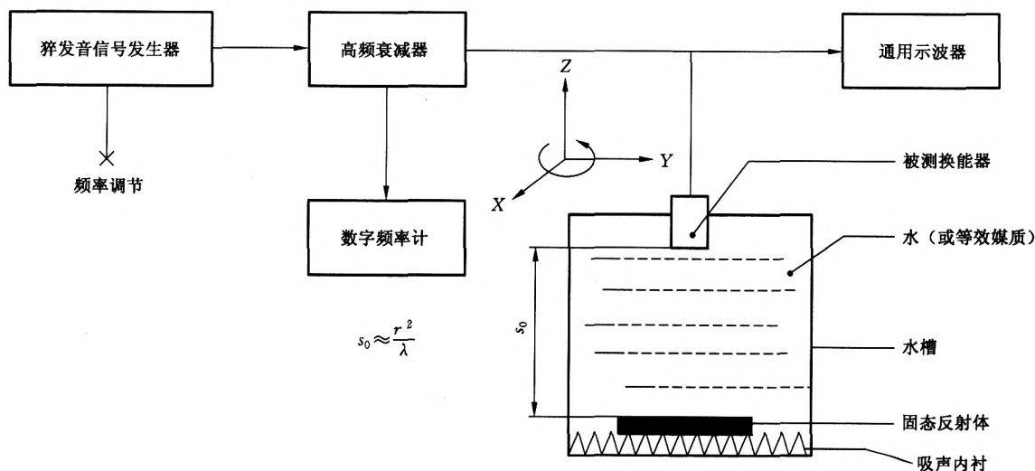
图 2 测量换能器频率特性和相对脉冲回波灵敏度级的原理图
