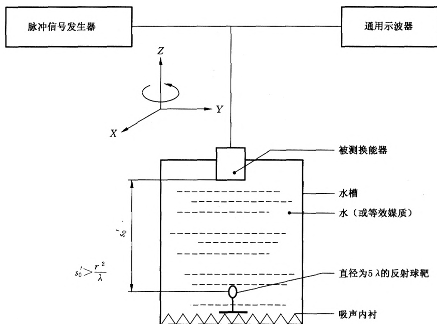
图 13 测量脉冲回波波束宽度的原理图
