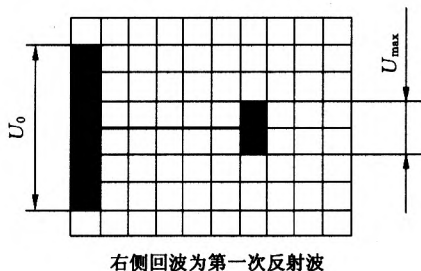
图 5 U_0 和 U_{\max} 在屏幕上的示意图
