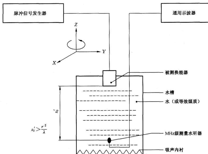
图 10 测量发射波束宽度的原理图
