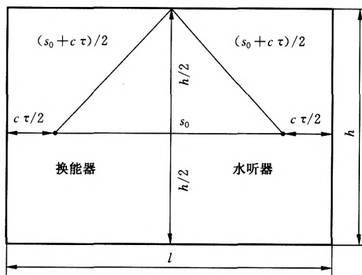
图 1 水槽尺寸
