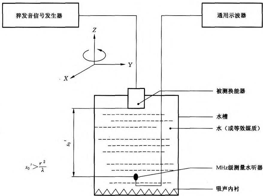
图 9 测量发射电压响应级的原理图
