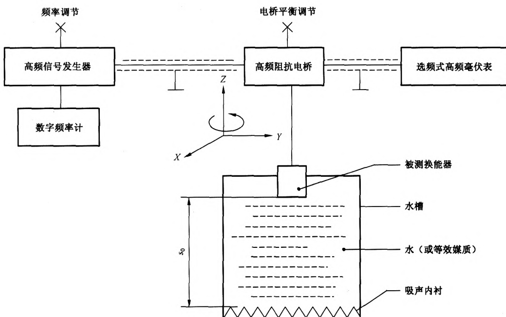
图 14 测量电阻抗的原理图
