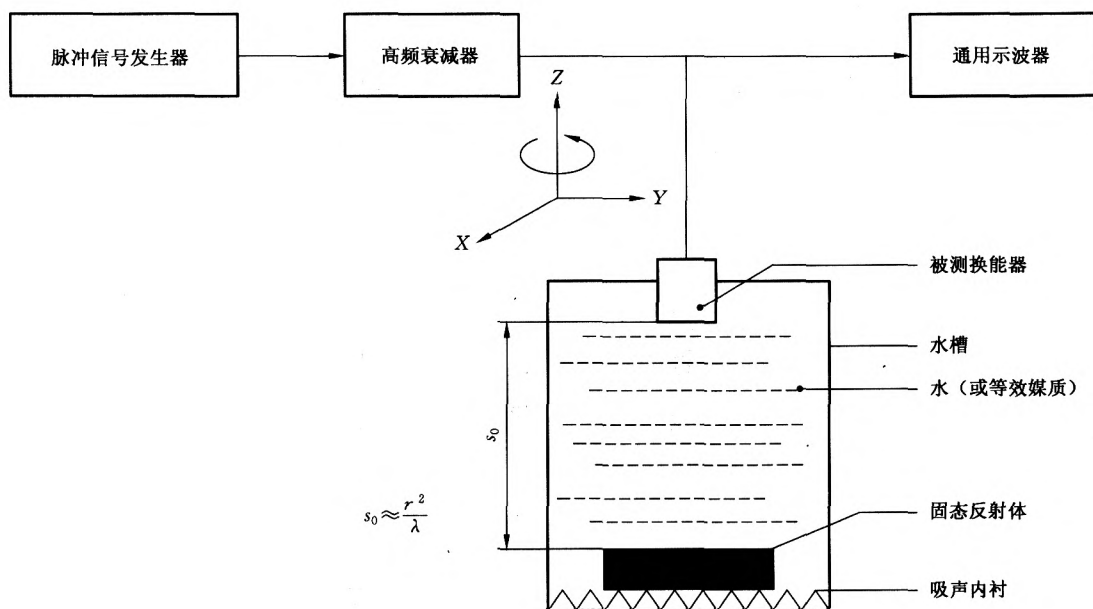
图7 测量回波脉冲宽度的原理图
