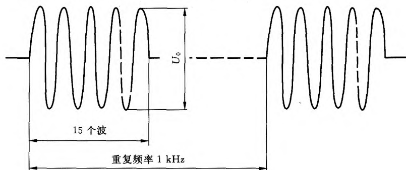
图 3 猝发音信号波形参数
