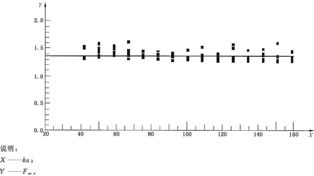
图 E.1 ka 乘积介于 40~160 之间时,转换因子 F_{\text{ac}} 和 ka 乘积间的函数关系
