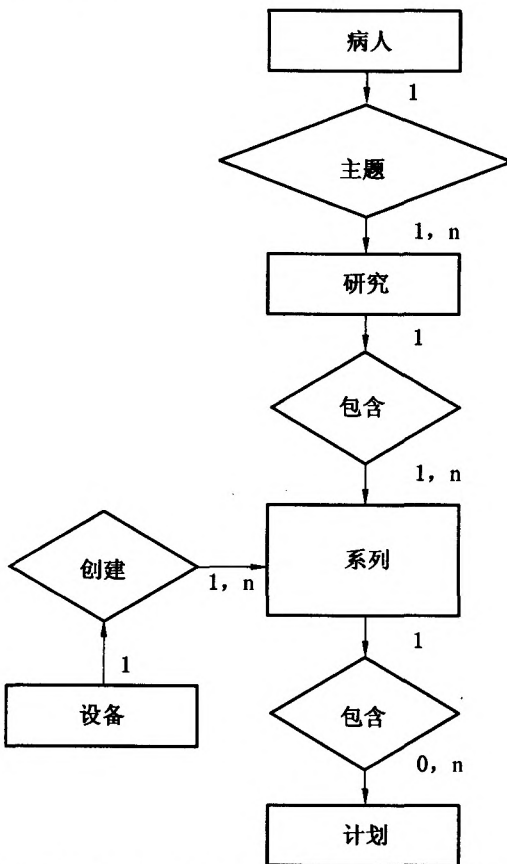
图 A. X-1 DICOM RT 计划 IOD 信息模型
