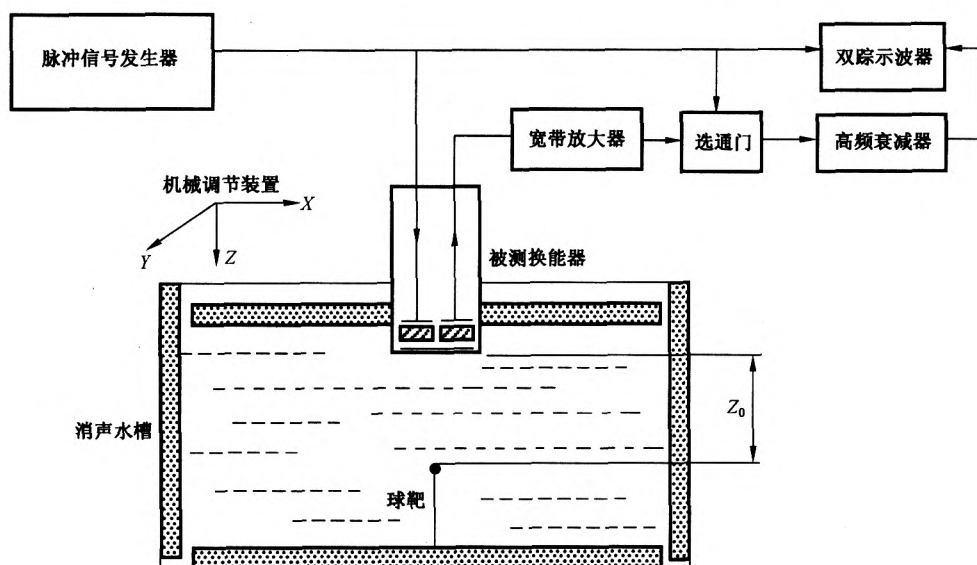
图3 换能器波束特性测量原理图
