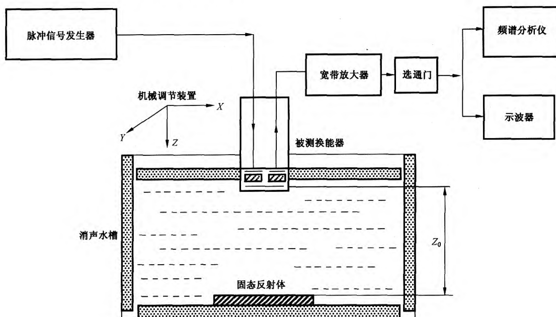
图 2 频谱分析法测试原理图
