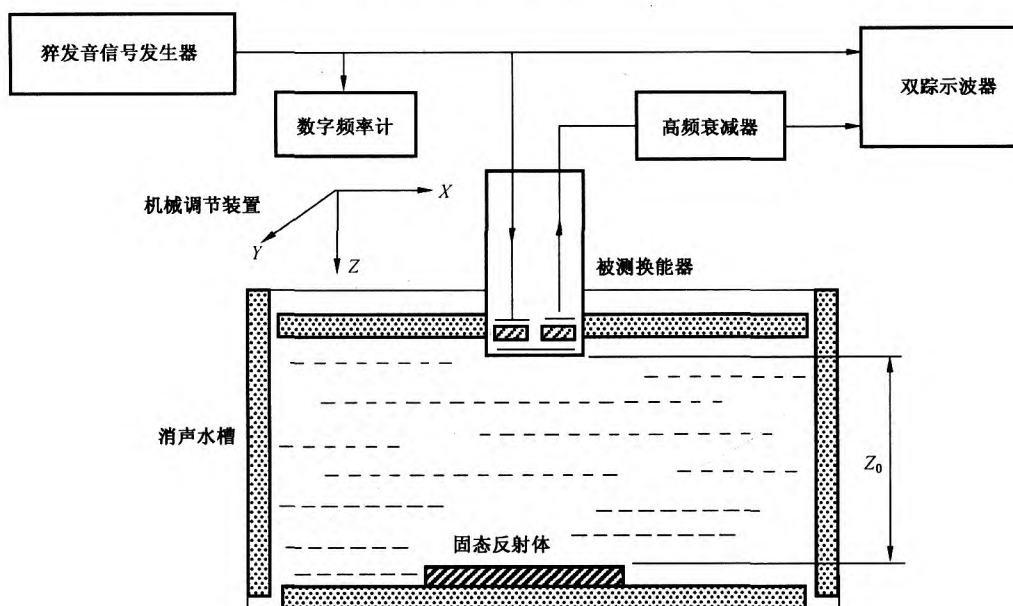
图 1 猝发音法测试原理图
