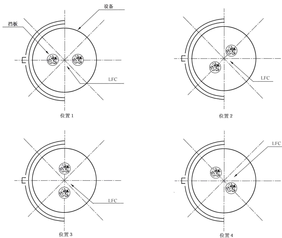
图 201.109 测量双遮板无影率时的双遮板四个不同位置
