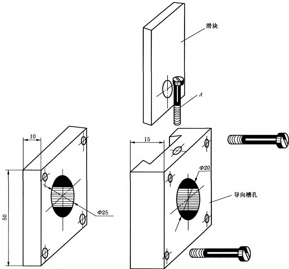
图 5 剪切粘接强度试验装置
