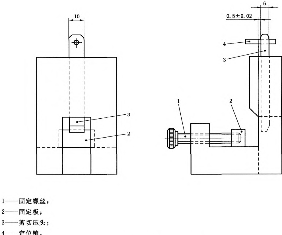
图 4 剪切粘接强度试验装置
