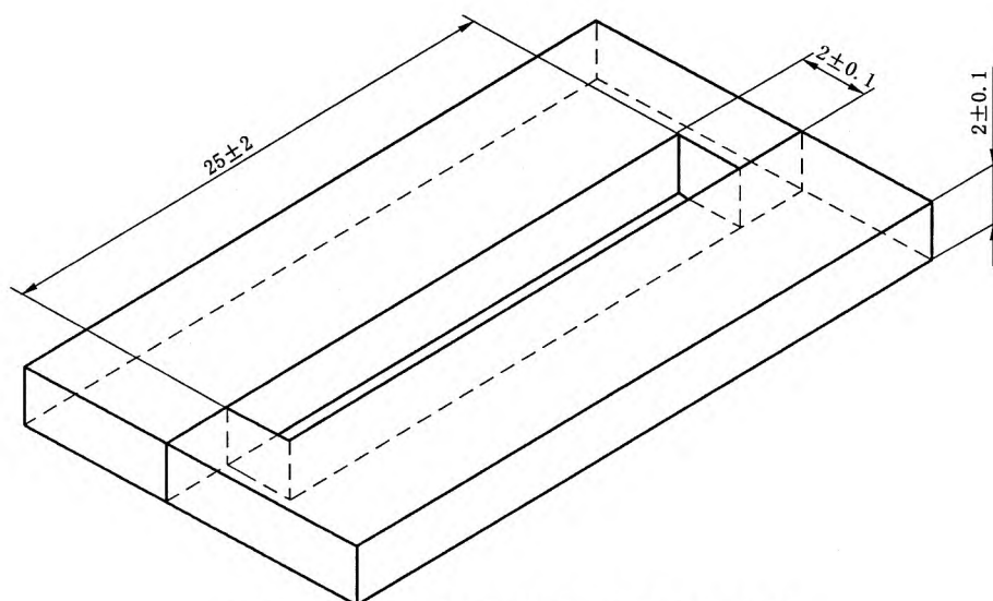
图 3 挠曲强度试样制样用不锈钢对开模具
