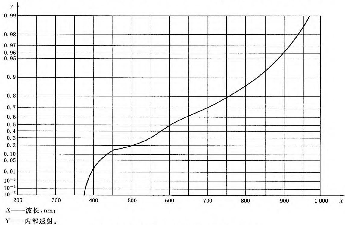
图 1 颜色转换滤光片的内部透射率(7.3.1.1)
