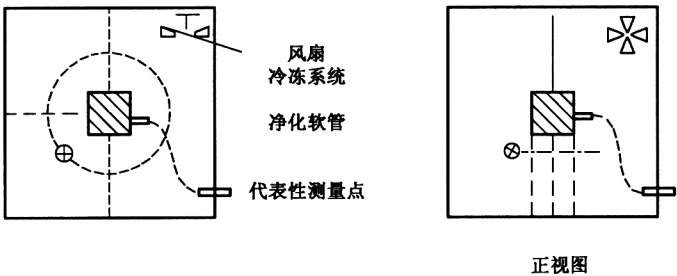
图 2 标准检测室
