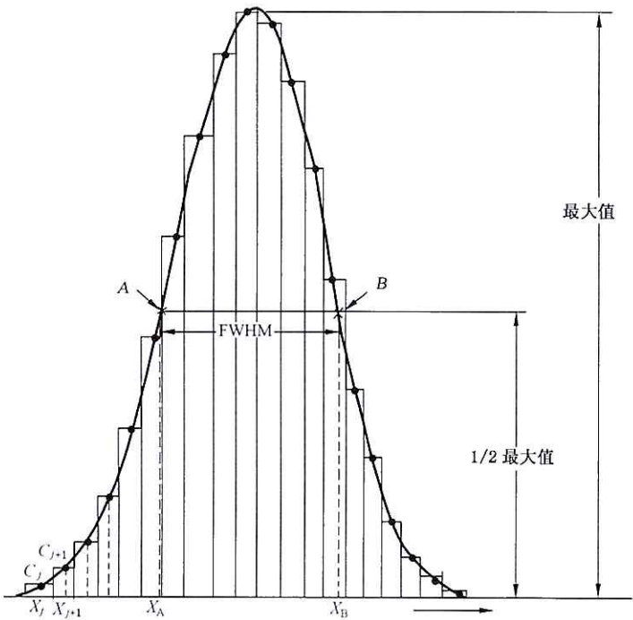
图 6 横向分辨率显示图
