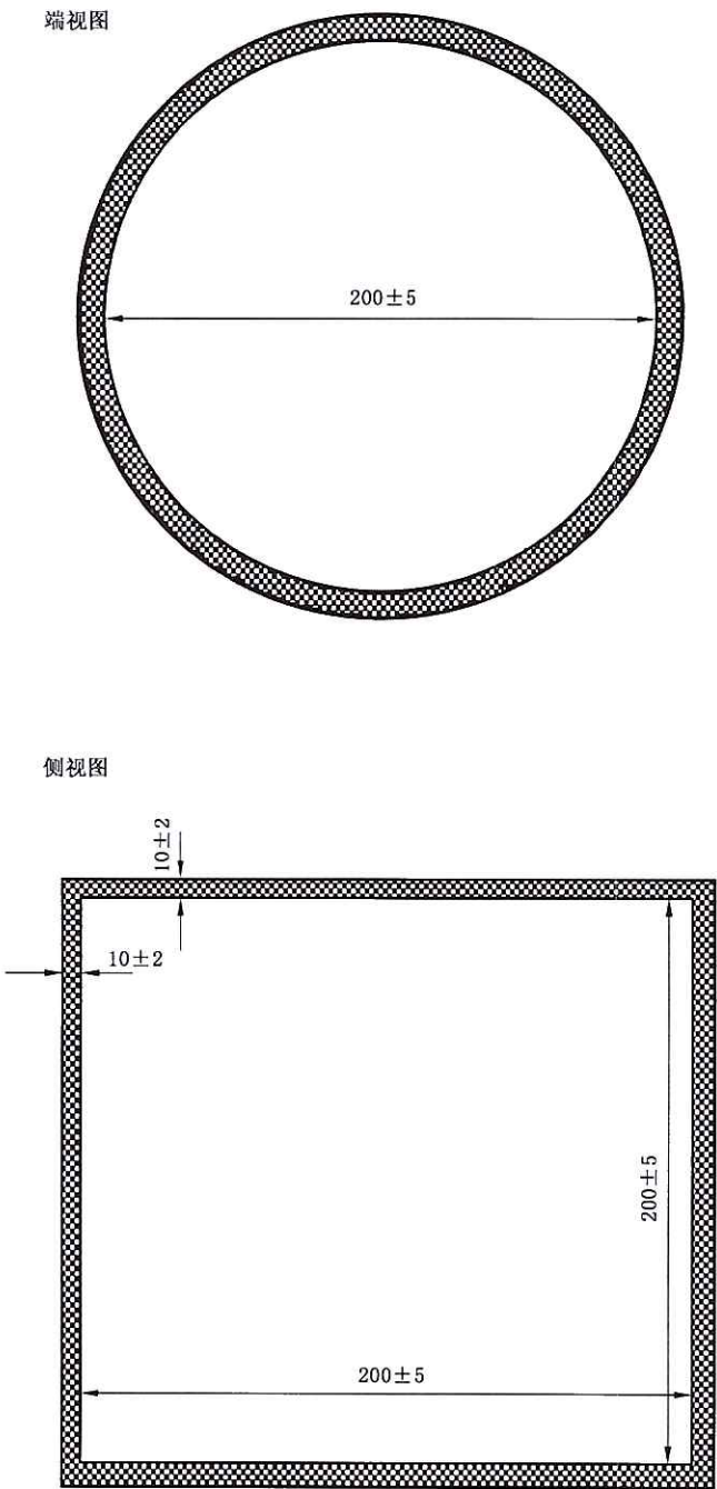
图 E.4 体积灵敏度测试模型
