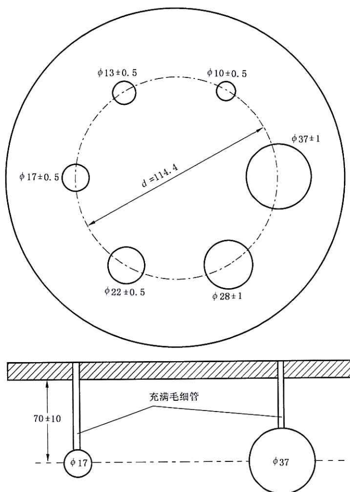
图3 手臂模体剖面图
