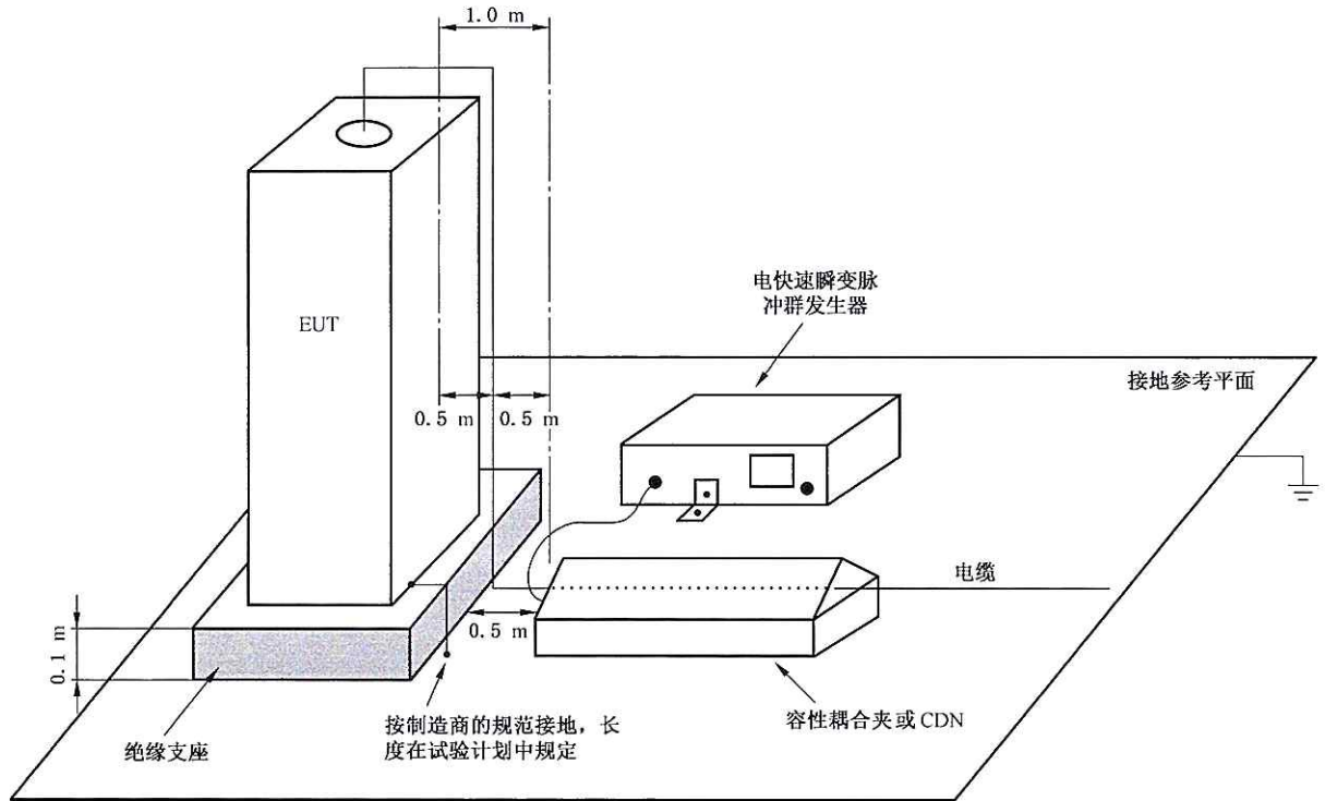
图 13 架高电缆的试验布置示例
