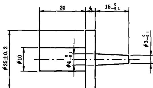
图 2B 试验针
