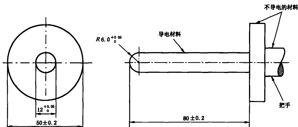
图 2C 试验探头
