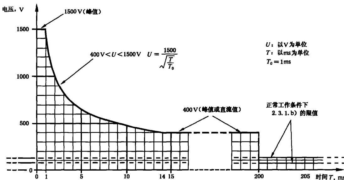
图 2D 单一故障后允许的最高电压
