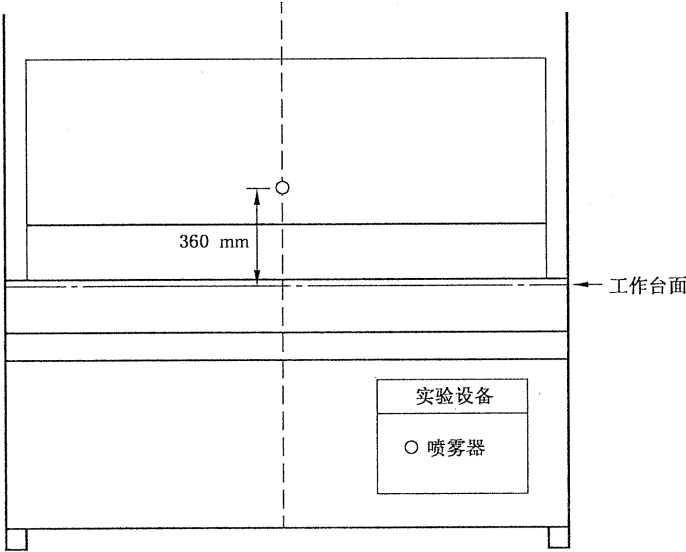
图 4 人员保护试验
