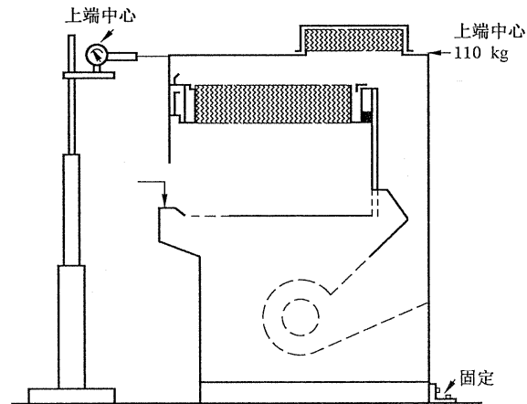
图 15 柜体抗变形试验(正面)
