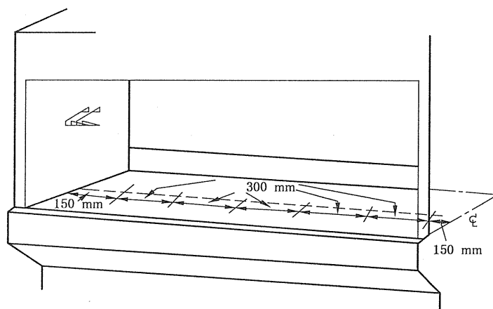
图 2 照度测试
