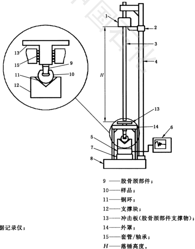
图 1 试验机示例
