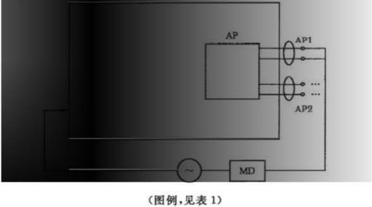
图 8 测量内部电源的医用电气设备应用部分漏电流的测量电路——直接法
