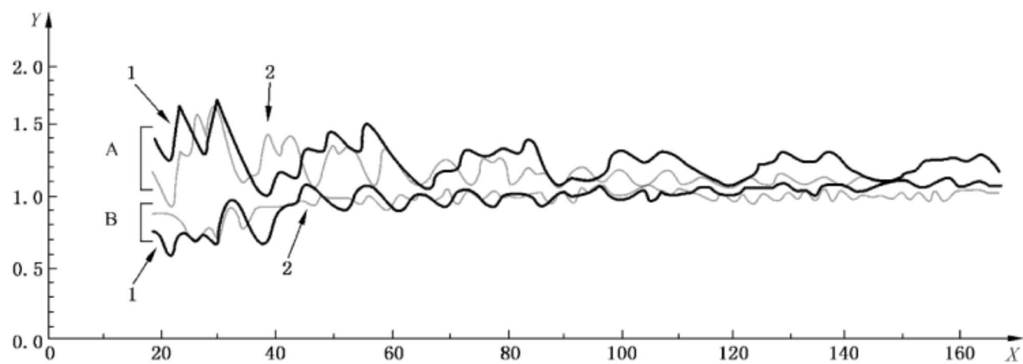
说明： X —— ka ； Y —— 归一化的波束横截面积(A 遵循 FDA 标准,B 遵循 IEC 标准 1 在 z=5\text{ mm} 处,2 在 z=2a 处,其中 a 为超声换能器有源元件的几何半径)。 注：在与治疗头为 5\text{ mm} 和 2a 的距离上进行计算。
