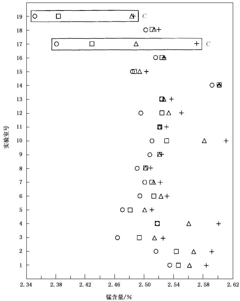
图 B.5 铁矿石中的锰含量:水平 5 的测试结果
