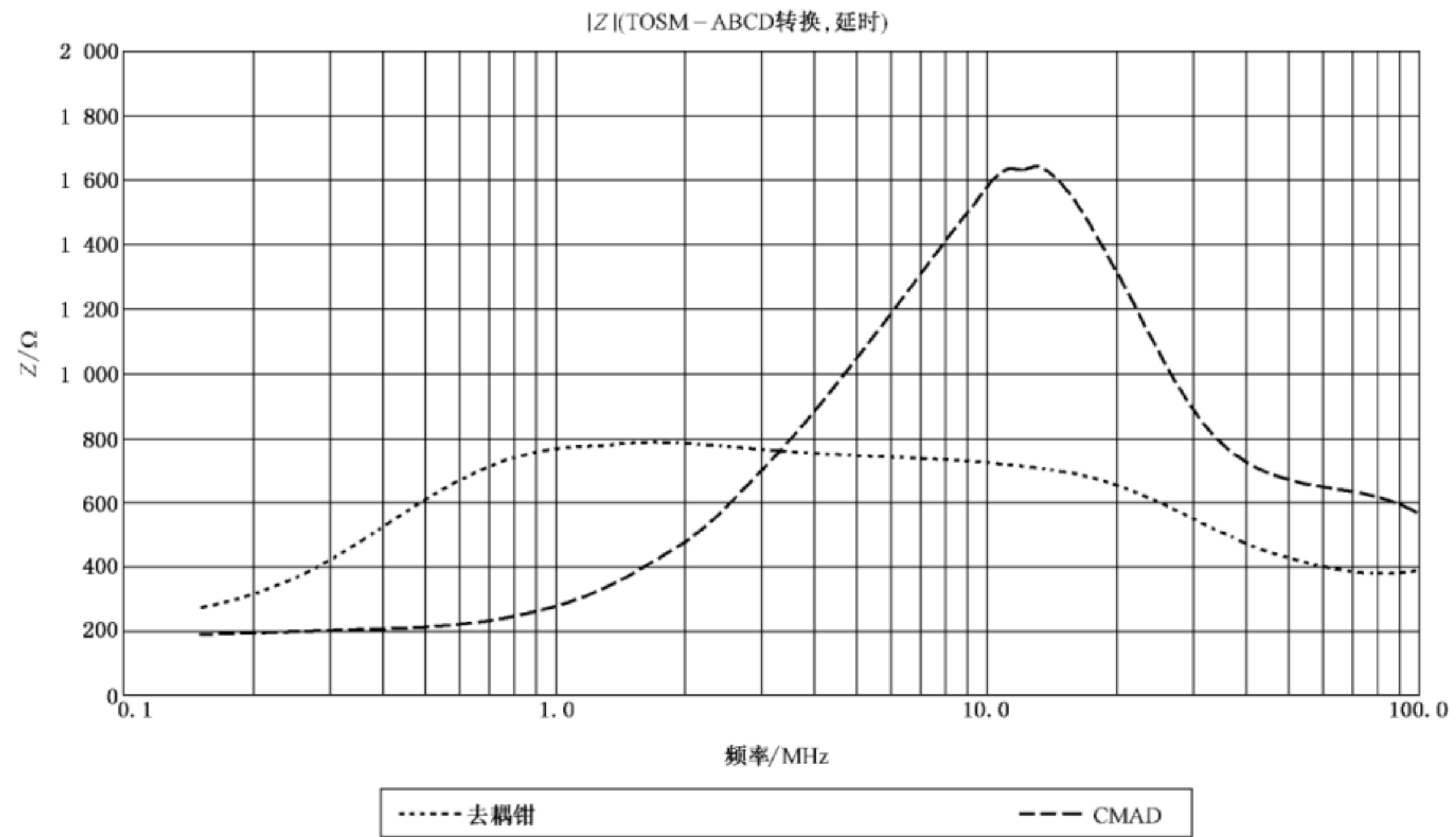
图 A.13 去耦钳阻抗的典型实例
