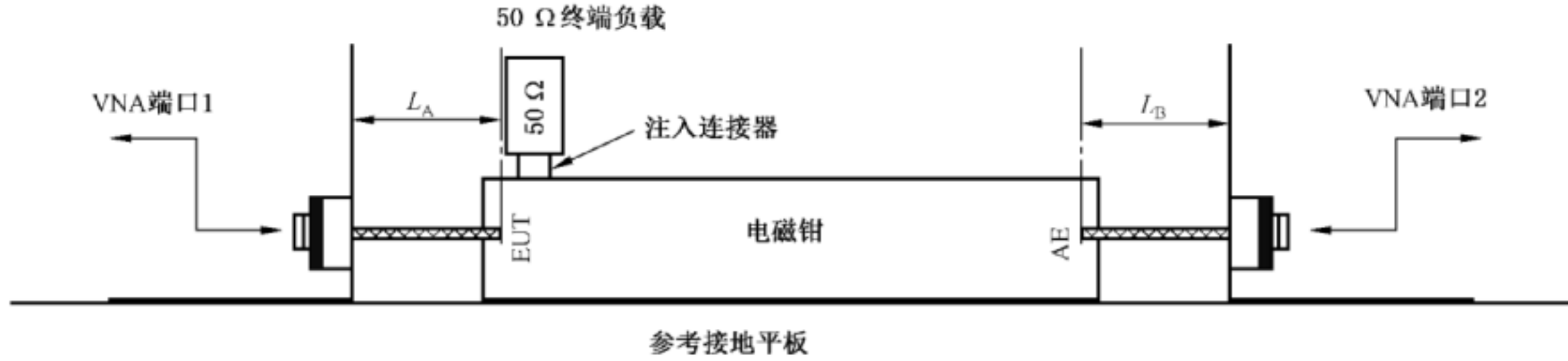
图 A.6 阻抗/去耦系数测量布置
