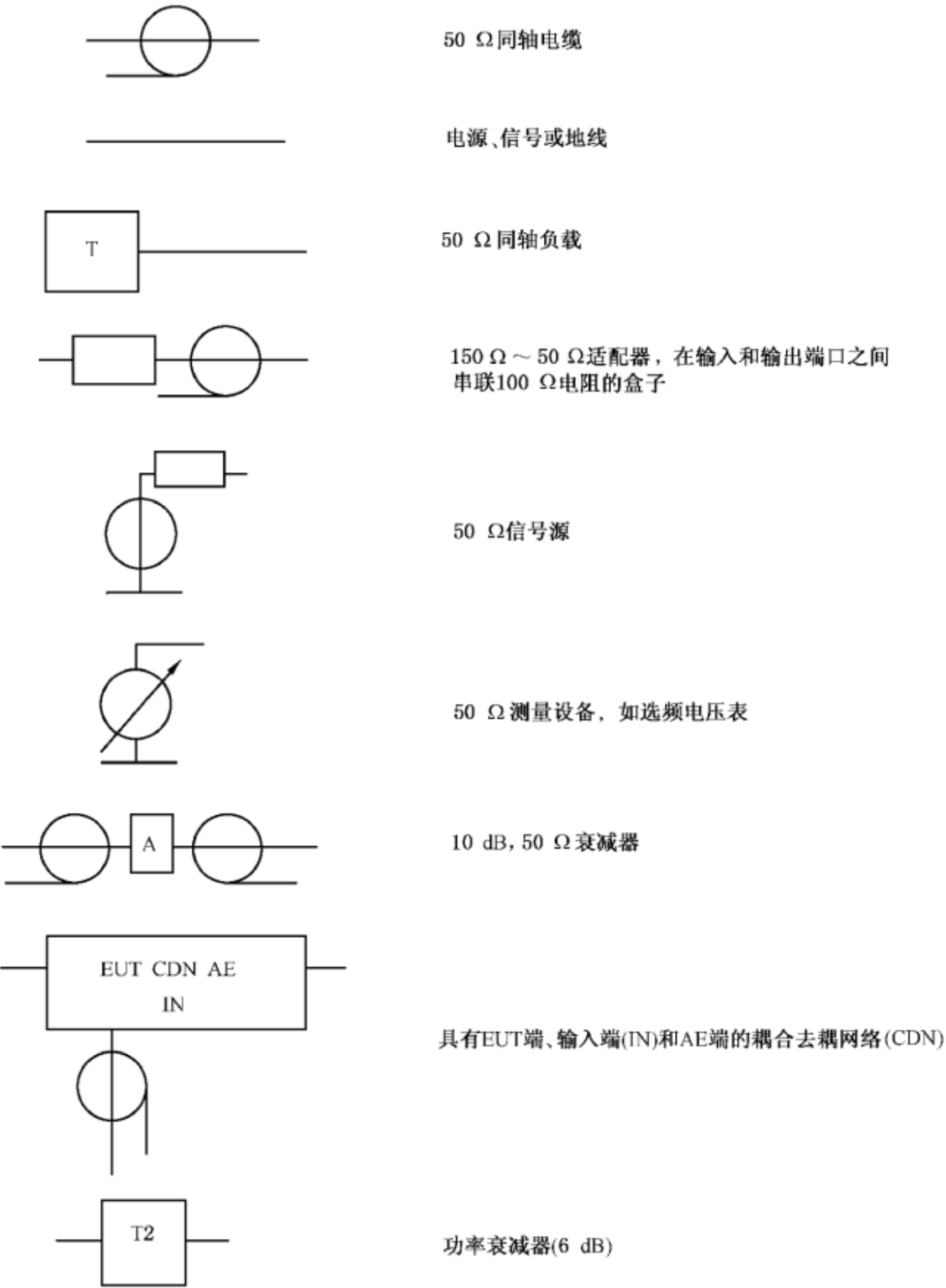
a) 用于测量配置图中的符号清单
