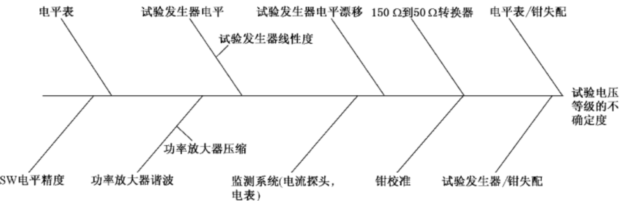
图 G.3 使用电流钳对试验电压电平的影响量示例
