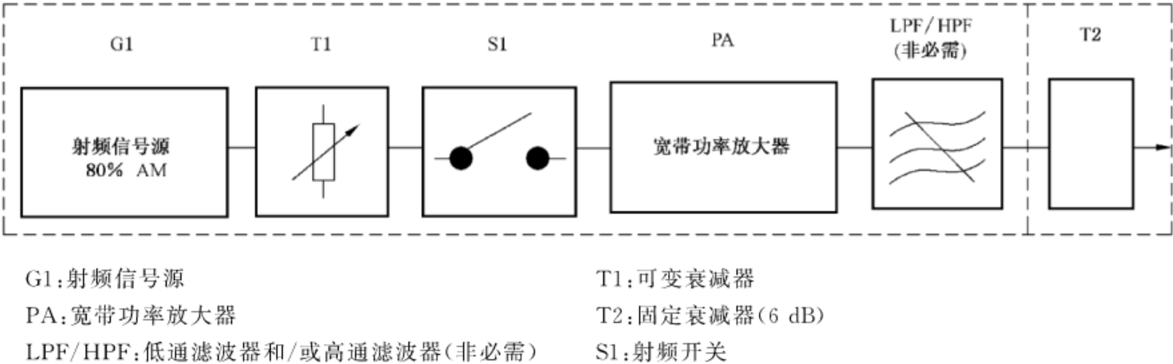
图 3 试验信号发生器的配置
