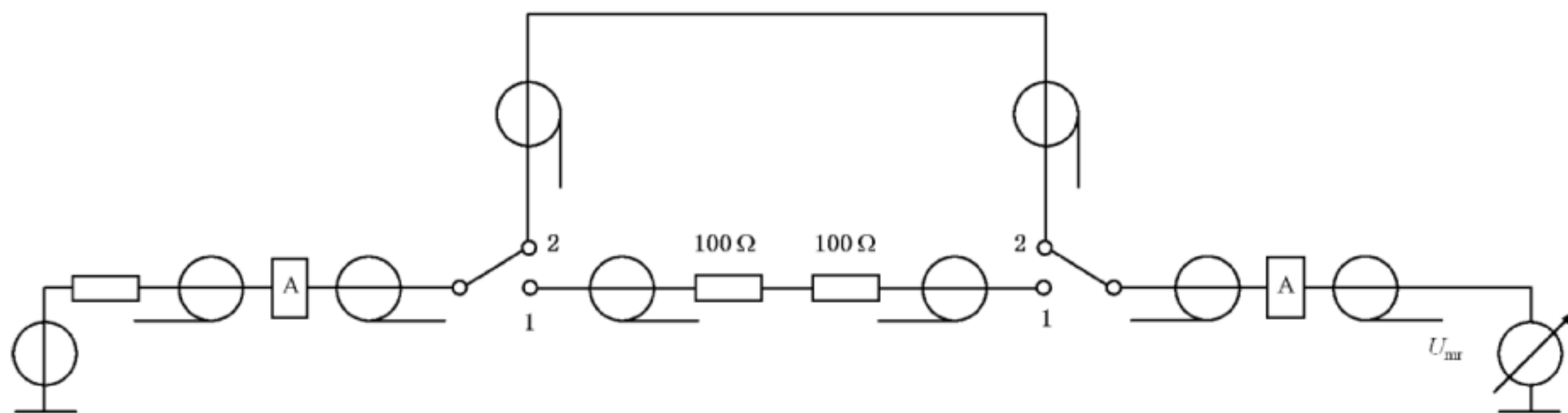
b) 验证耦合/去耦装置 Z_{ce} 的配置原理图
