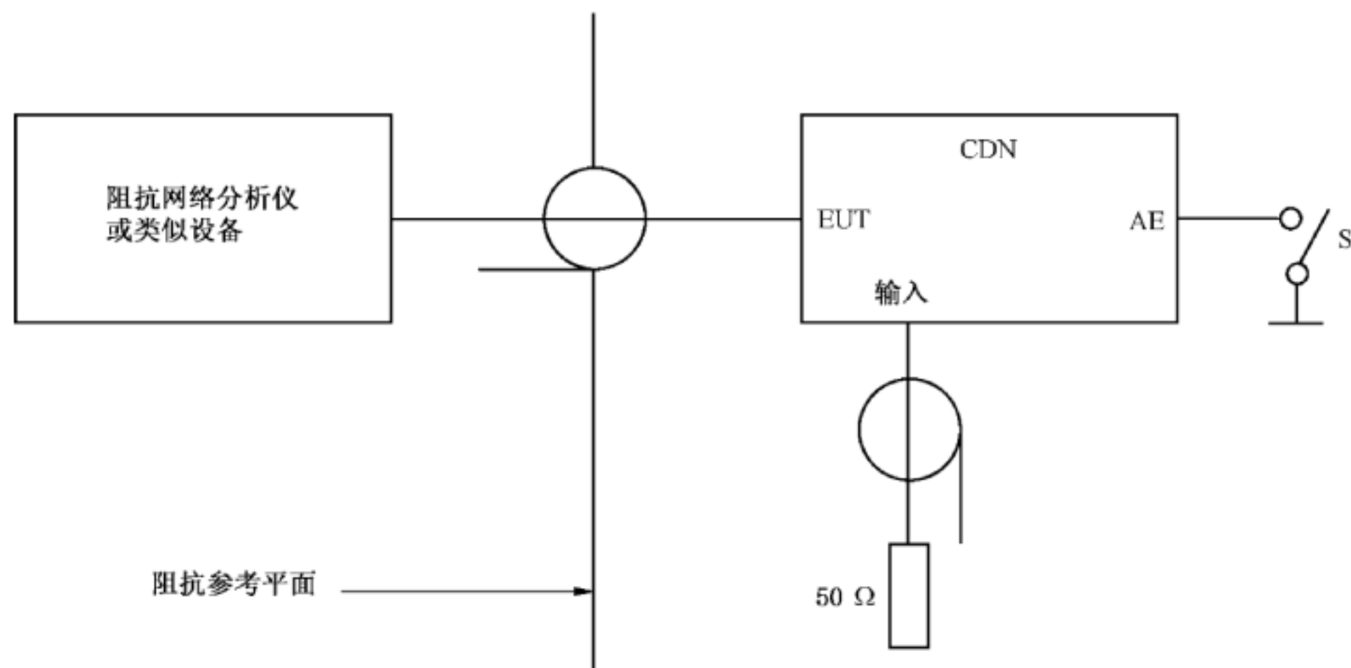
a) 验证耦合/去耦装置阻抗特性的配置示例
