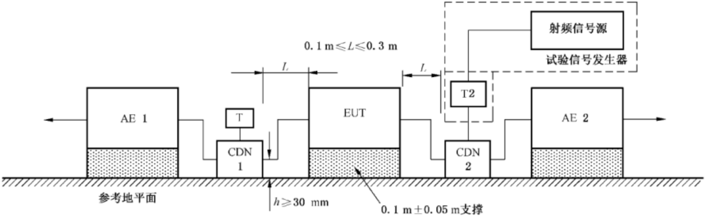
使用 CDN 的抗扰度试验布置示意图
