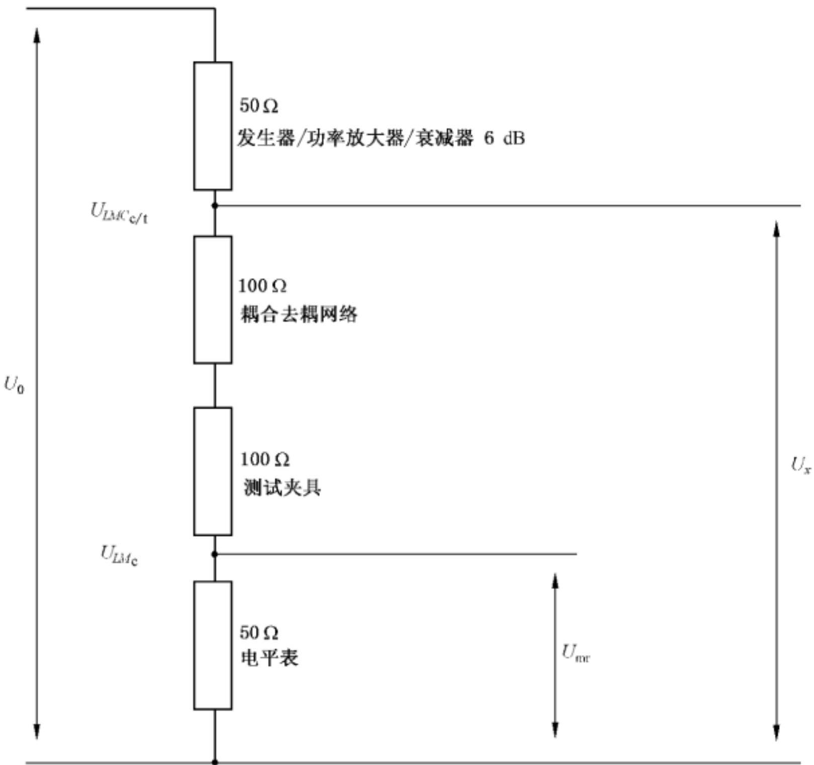
图 G.5 电平调整电路示意图
