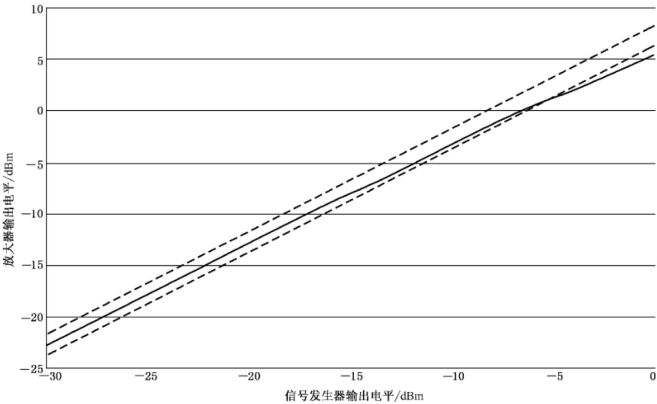
图 J.2 线性特性
