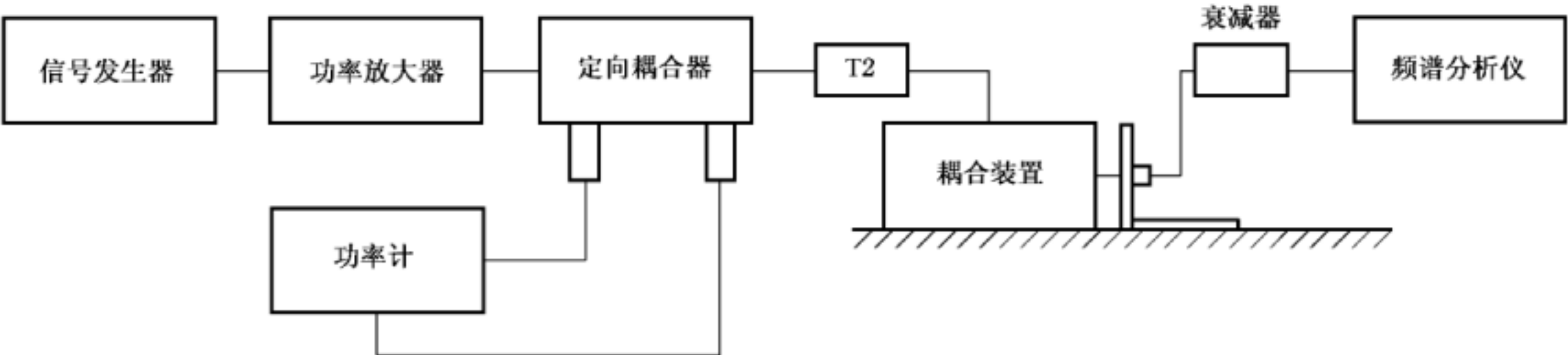
图 J.1 放大器的线性测量的布置
