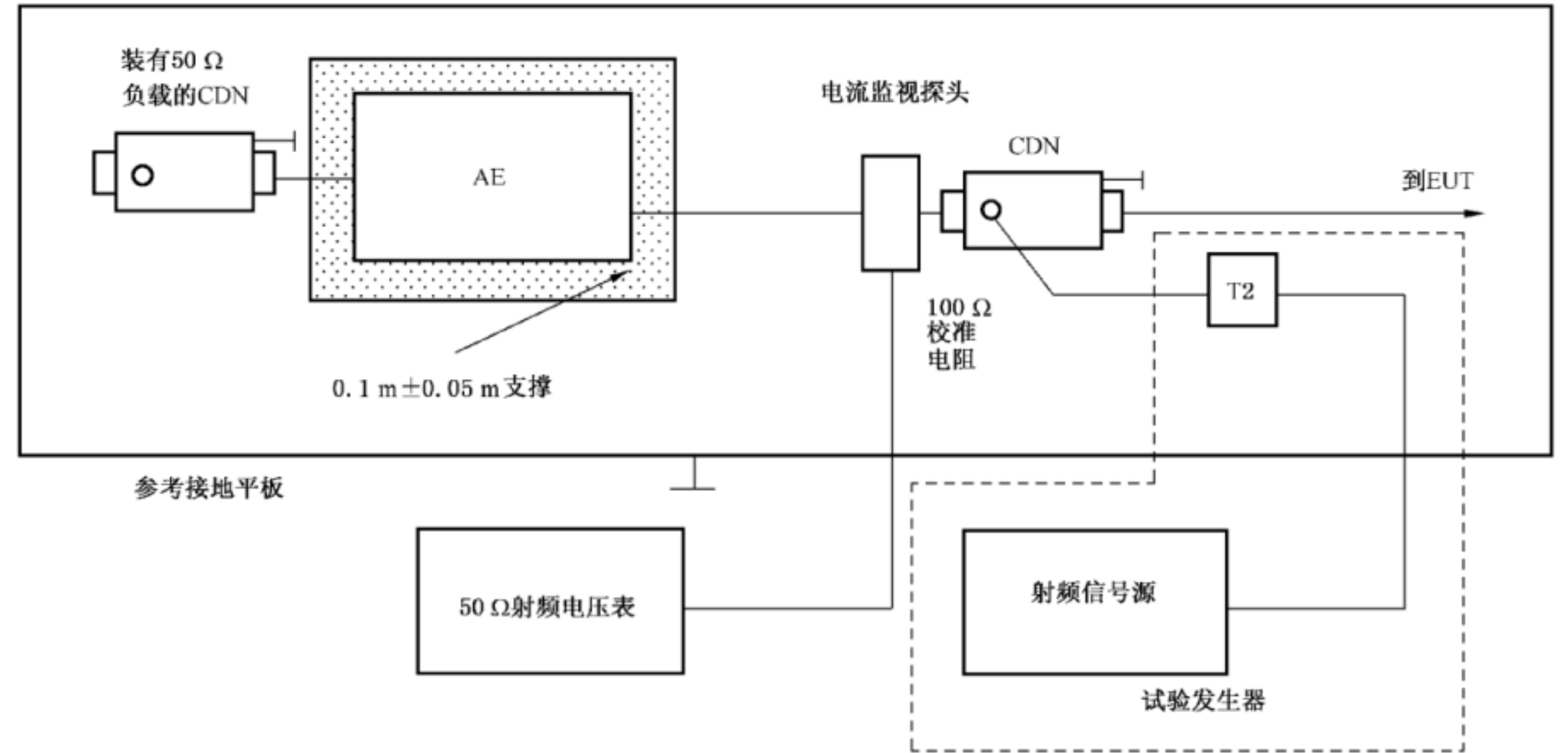
图 H.2 使用电流探头测量阻抗
