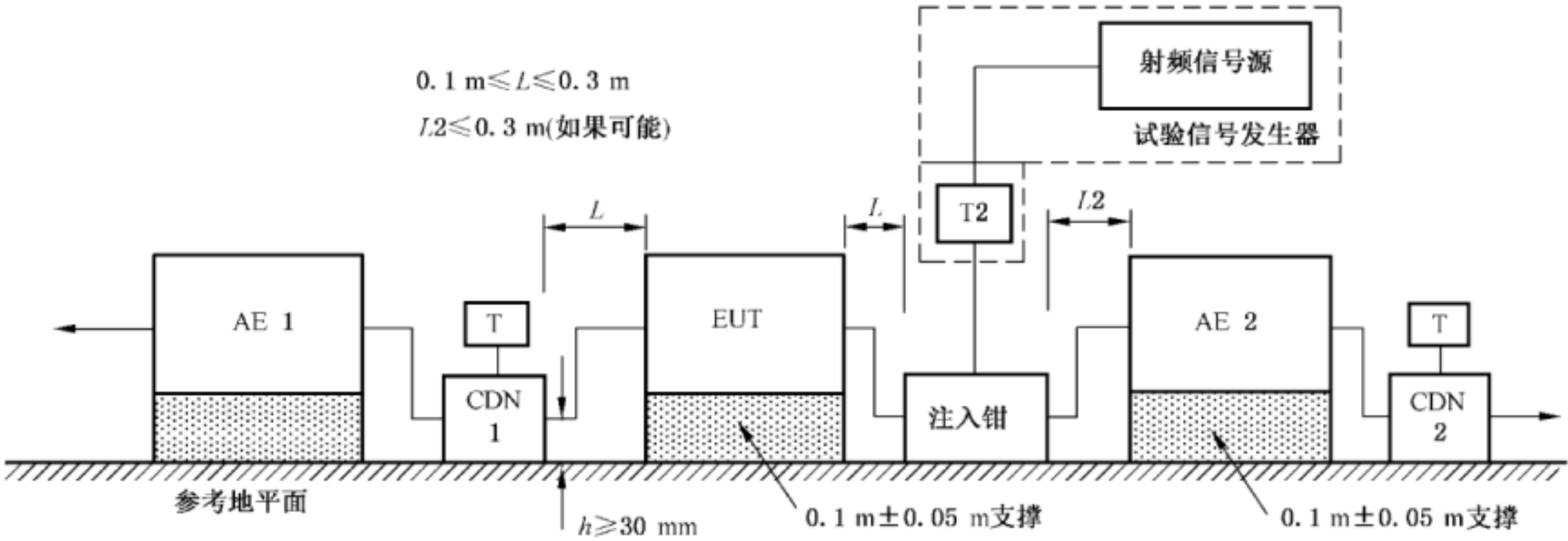
使用 CDN 的抗扰度试验布置示意图
