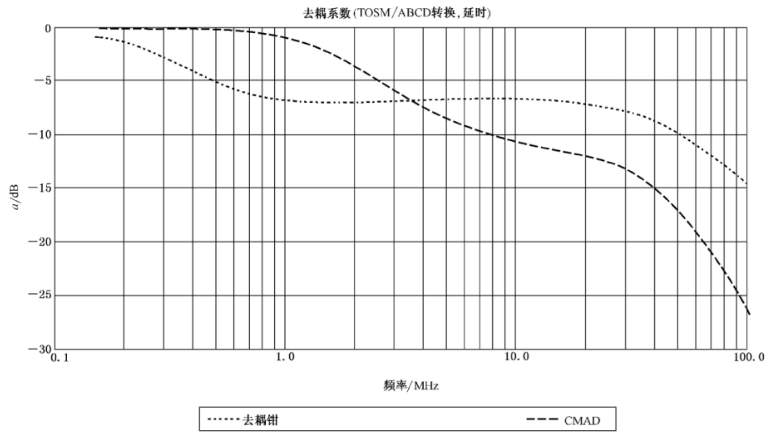
图 A.14 去耦系数的典型实例
