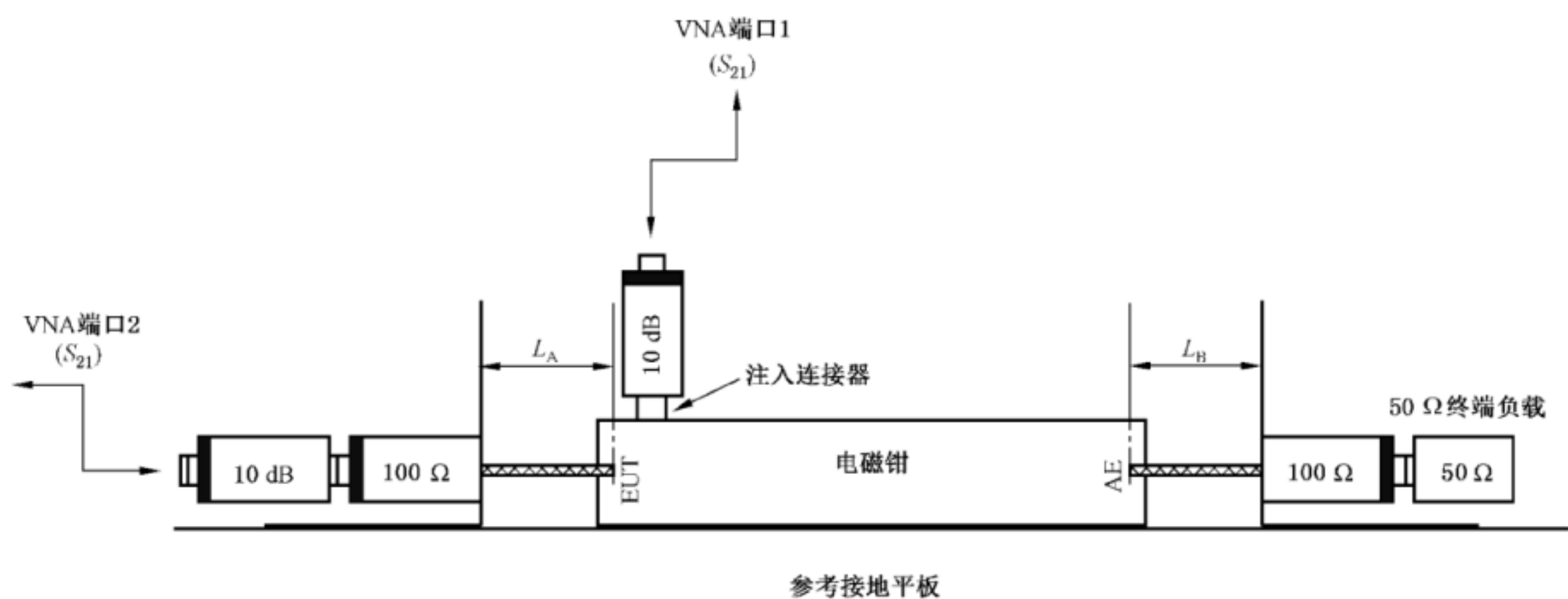
图 A.10 S_{21} 耦合系数测量布置
