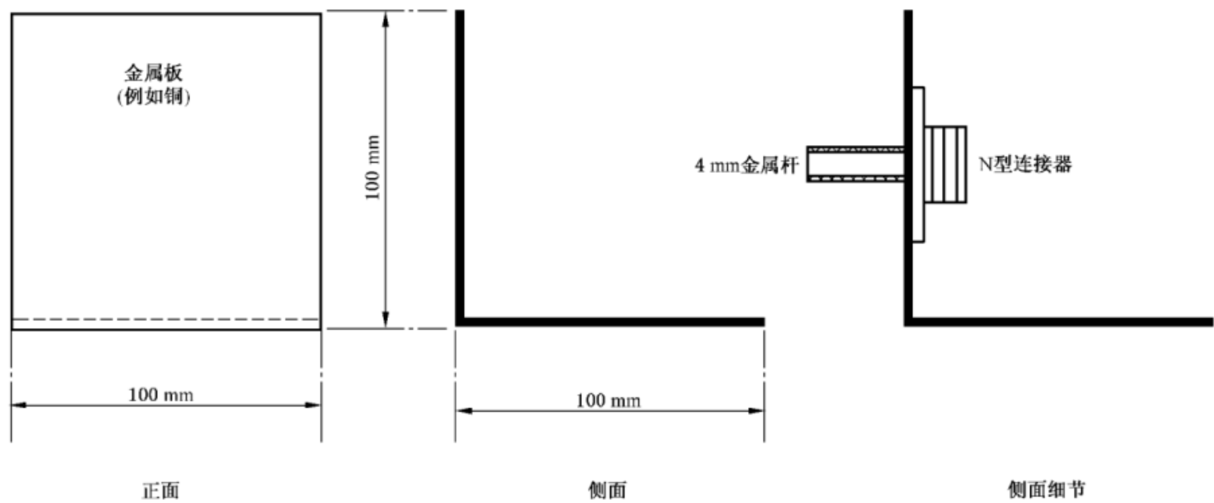
图 A.3 参考平面尺寸
