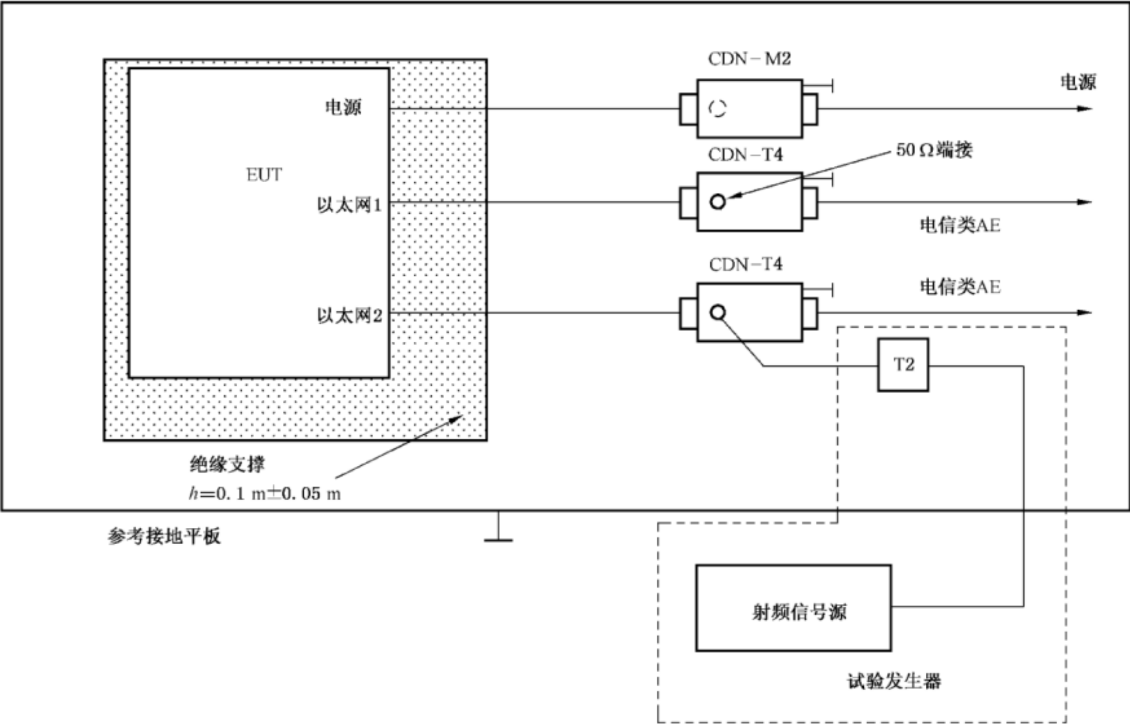
图 I.1 端口间注入试验布置的示例
