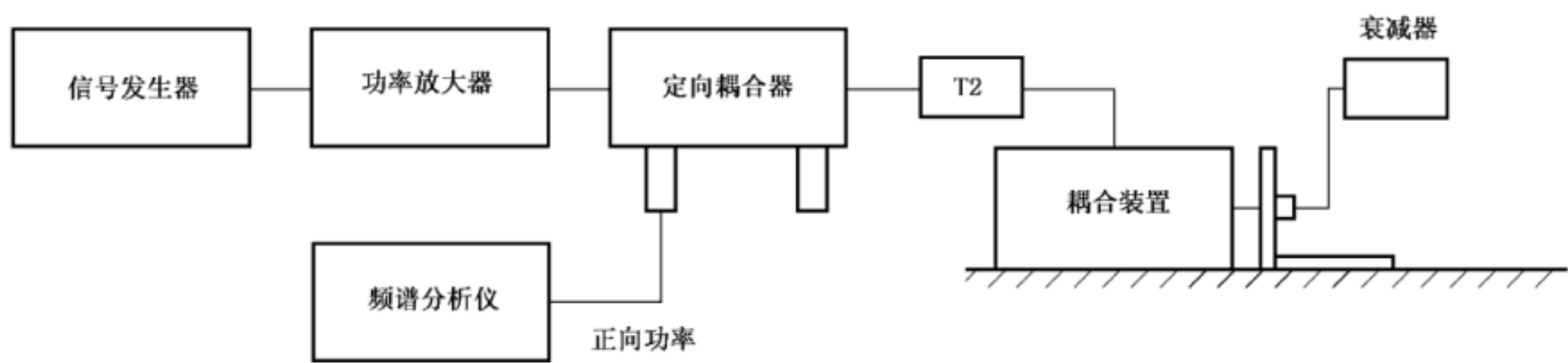
图 J.3 调制深度的测量布置
