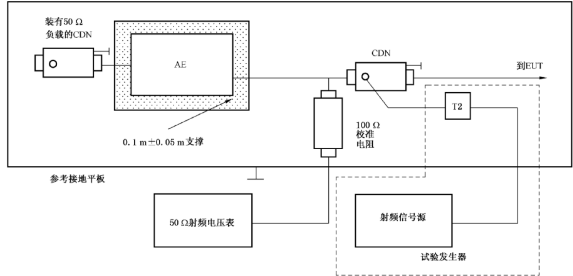
图 H.1 使用电压表阻抗测量框图
