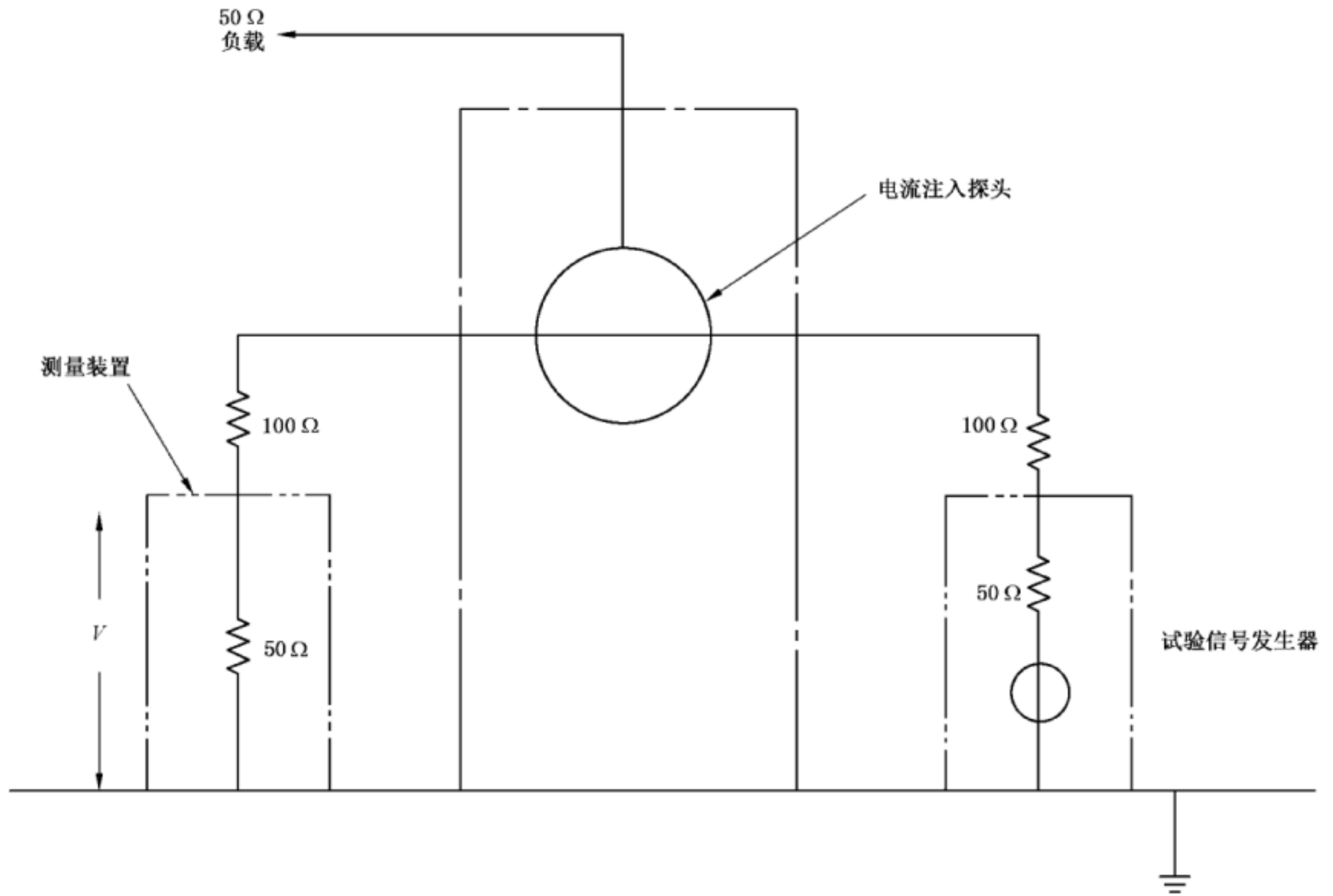
图 7 电流钳的性能评价电路示例
