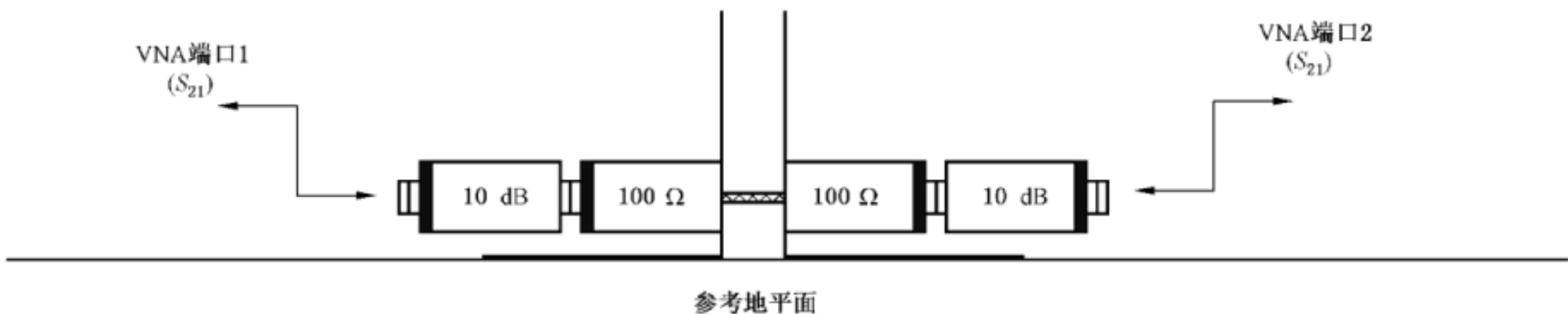
图 A.9 耦合系数测量的归一化布置
