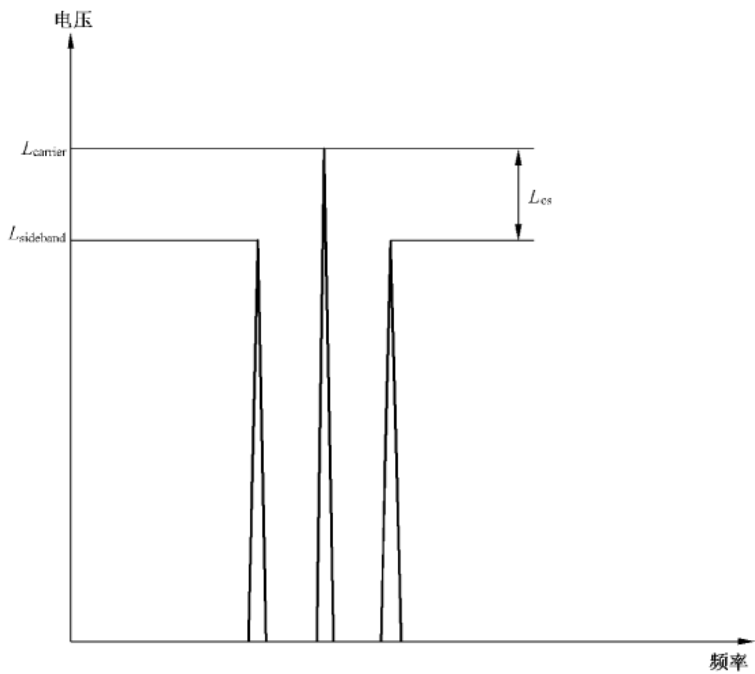
图 J.4 AM 调制信号的频谱示意图
