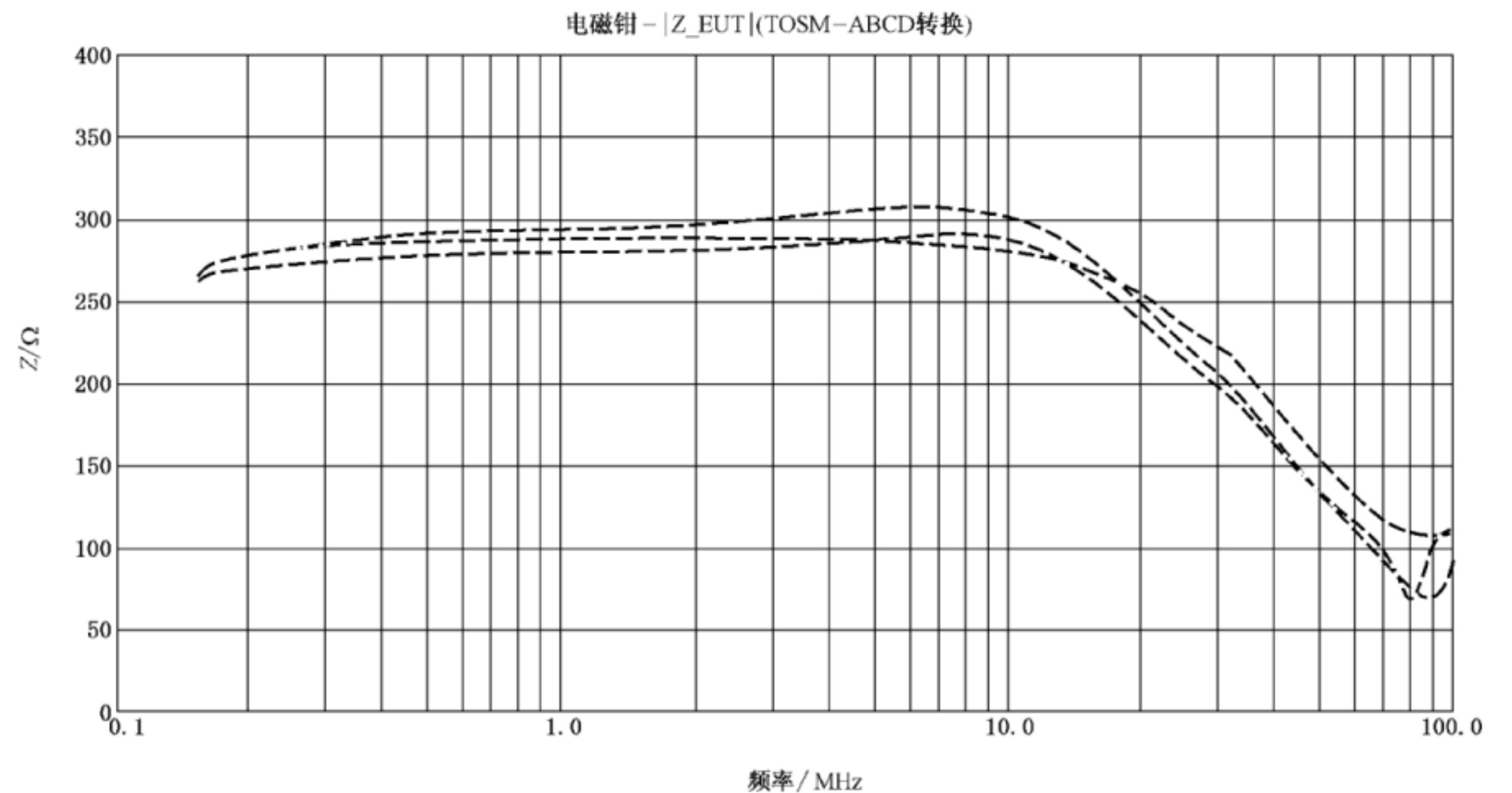
图 A.7 三种电磁钳阻抗的典型实例
