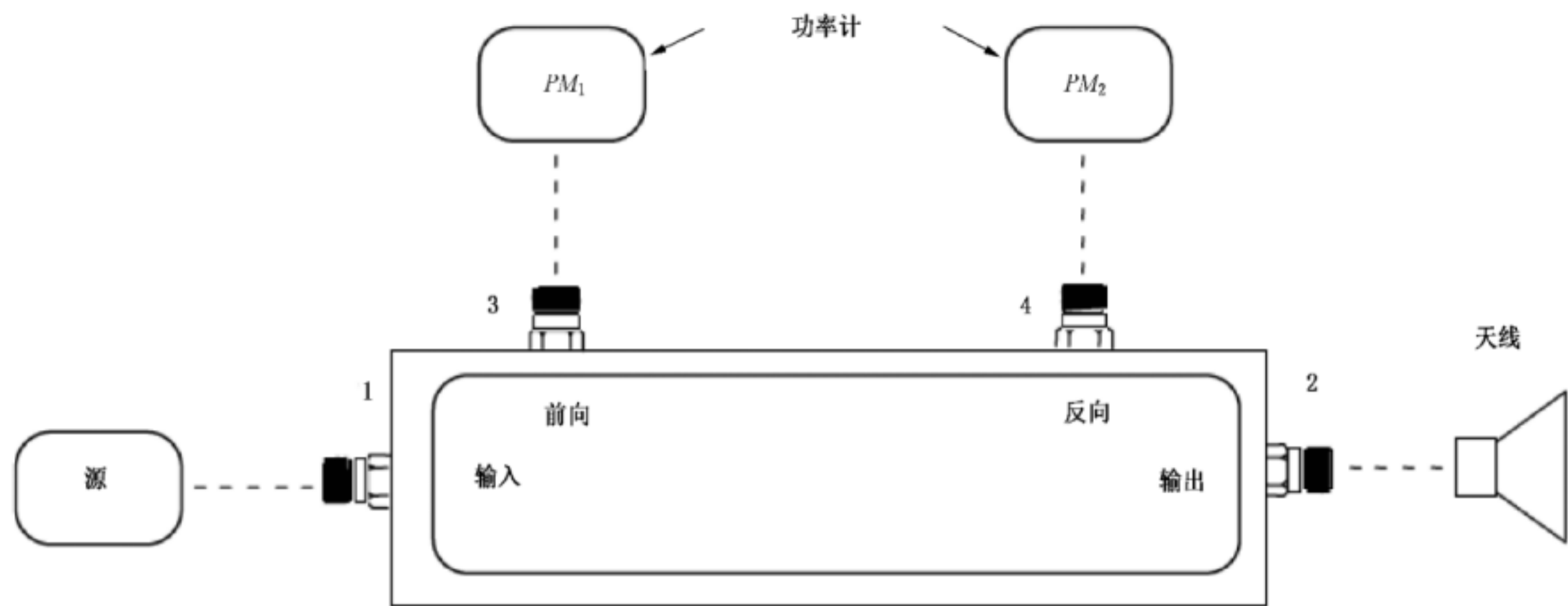
图 I.2 发射装置净功率测量配置
