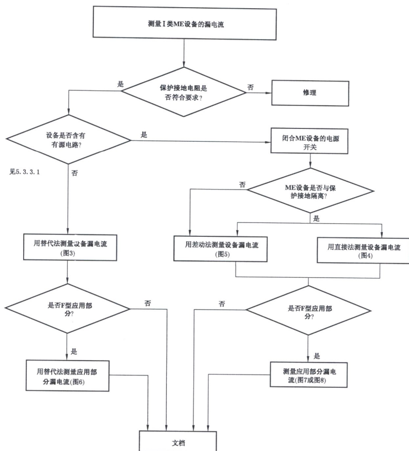
图 B.2 测量漏电流 (I 类 ME 设备)
