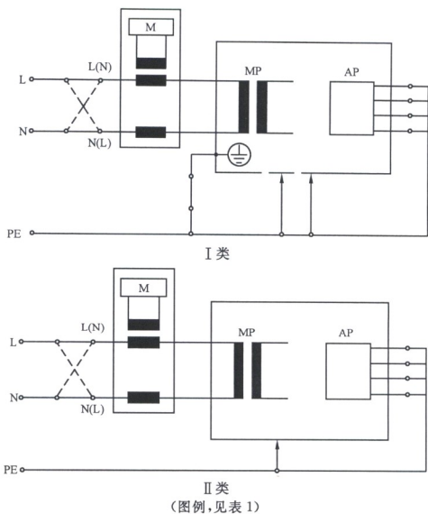
图 5 测量设备漏电流的测量电路——差值法
