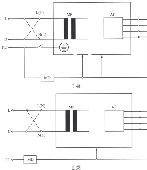
图 4 测量设备漏电流的测量电路——直接法
