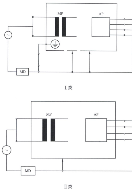
图 3 测量设备漏电流的测量电路——替代法
