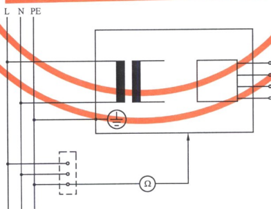
图 2 ME 设备或 ME 系统保护接地电阻的测量电路。ME 设备或 ME 系统因为功能原因无法从供电网中断开,或其与供电网有永久性连接
