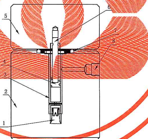
图 2 夹具与非透气硬质供试包装图示
